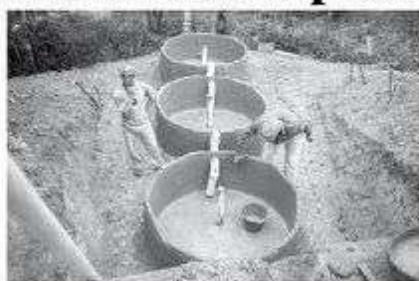
Construção da fossa em Monte Formoso
